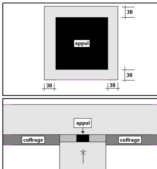
Fig.1 : Positionnement des appuis
